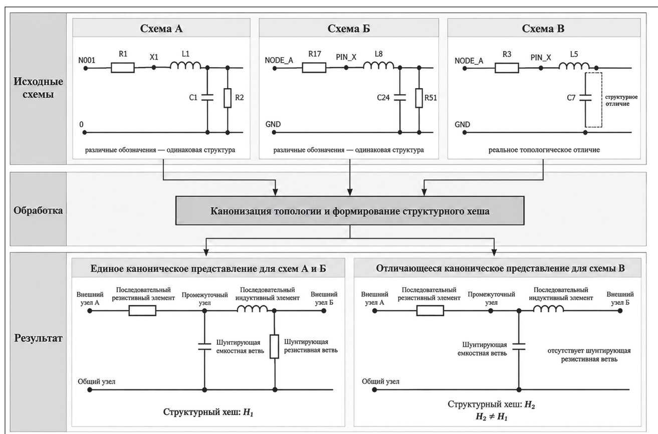
Рис. 2. Приведение структурно эквивалентных схем соединителя к единому каноническому представлению
