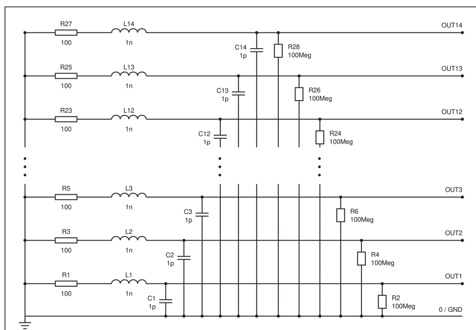
Рис.5. Графическая схема автоматически синтезированной модели 15-контактного соединителя
