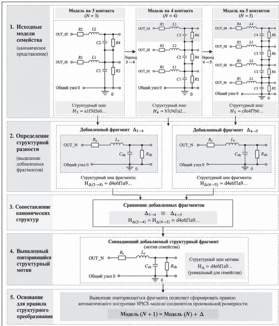
Рис.3 Выявление структурной закономерности по последовательности SPICE-моделей соединителя различной размерности
