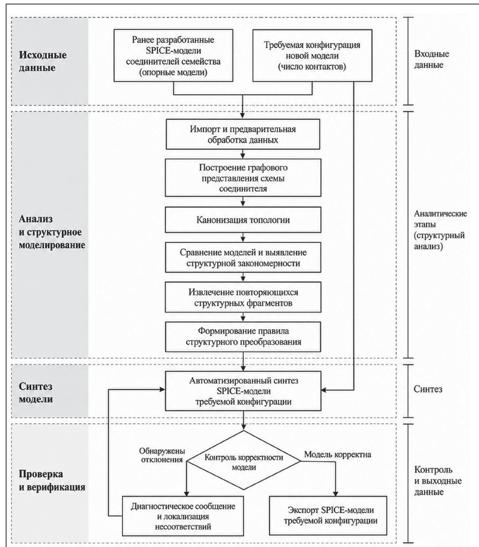
Рис. 1. Функциональная схема метода автоматизированного синтеза SPICE-моделей МЭС
