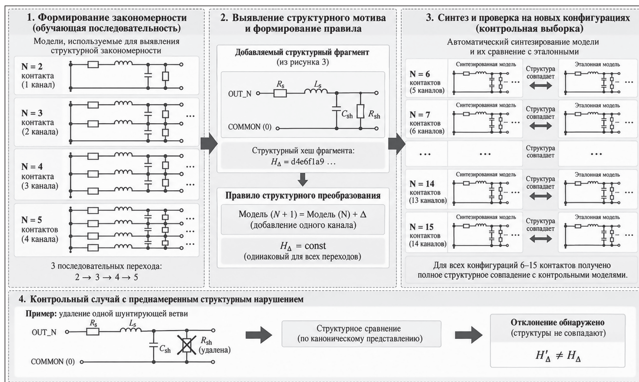
Рис. 4. Схема экспериментальной апробации метода автоматизированного синтеза SPICE-моделей соединителей
